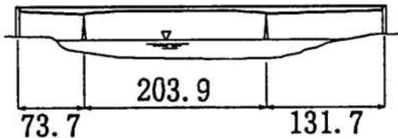
LSB50124,WEISENAU,,
