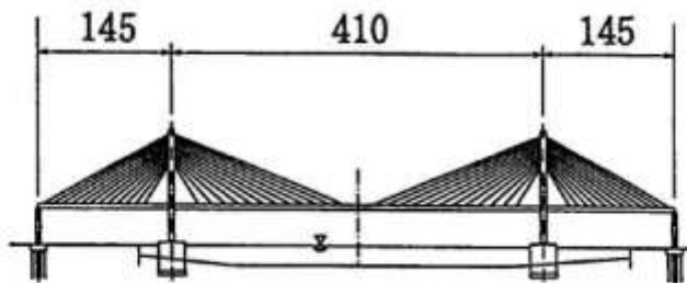
LSB20119, MEIKO-HIGASHI, 名港東大橋
