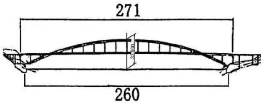
LSB30126,SAIGO,西郷大橋
