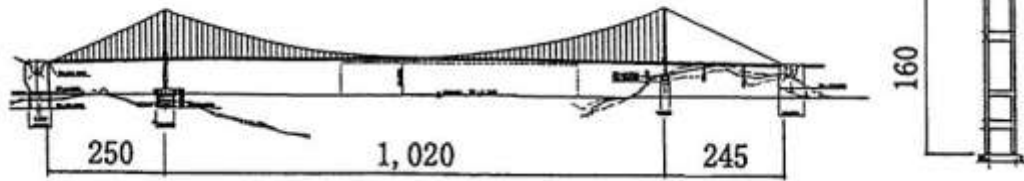
LSB10115,KURUSHIMA-II,来島第二大橋
