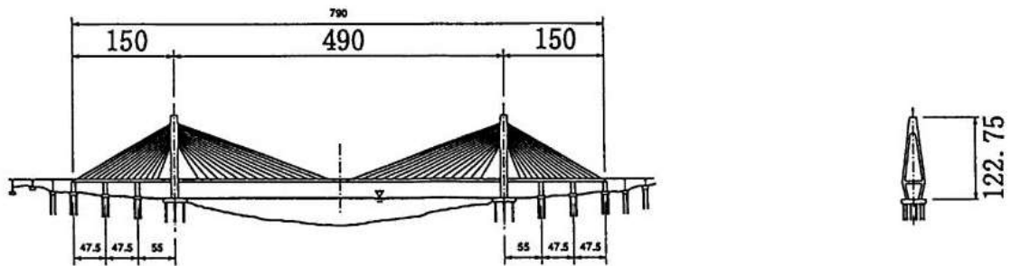
LSB20107,IKUCHI,生口橋
