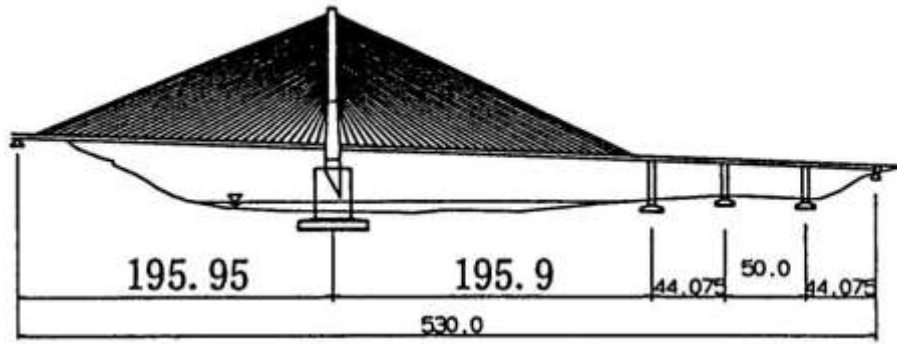
LSB20249,CHICHIBU-KOUEN,秩父公園橋
