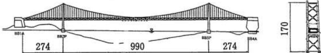
LSB10118,KITA-BISAN-SETO,北備讃瀬戸大橋
