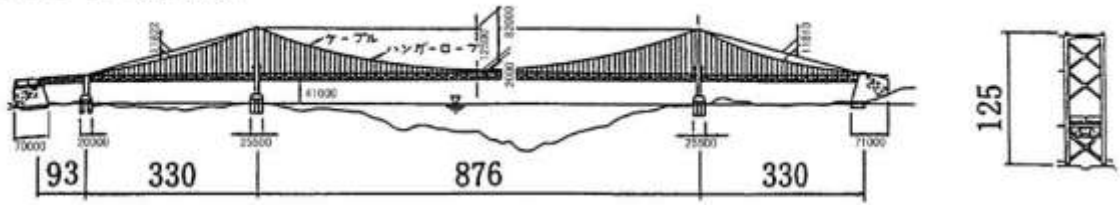
LSB10123, OHNARUTO, 大鳴門橋
