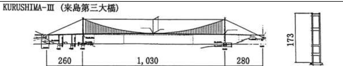
LSB10114, KURUSHIMA-III, 来島第三大橋
