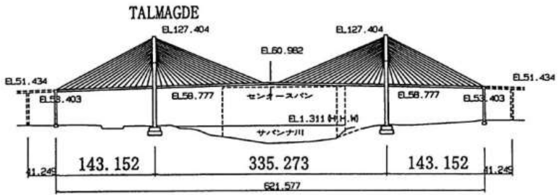
LSB20213,TALMAGDE,
