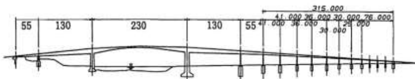
LSB50308,URATO,浦戸大橋,
