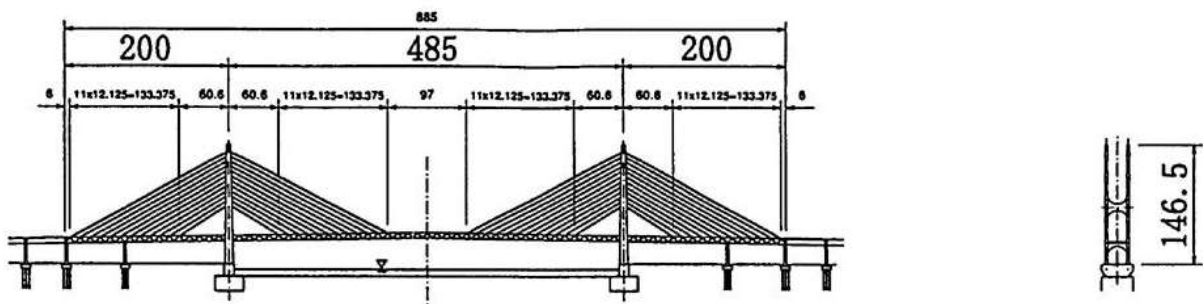
LSB20108,HIGASHI-KOBE,東神戸大橋
