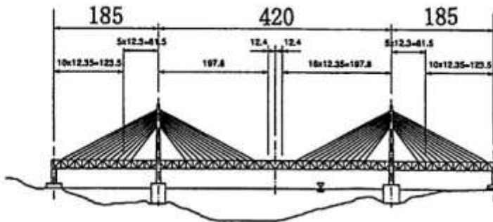
LSB20118, HITSUISHI-JIMA, 櫃石島橋
