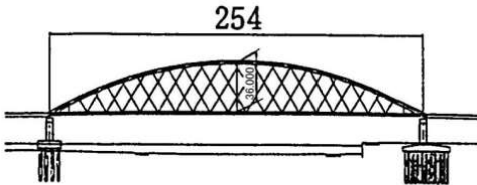
LSB30132,SHIN-HAMADERA,新浜寺大橋
