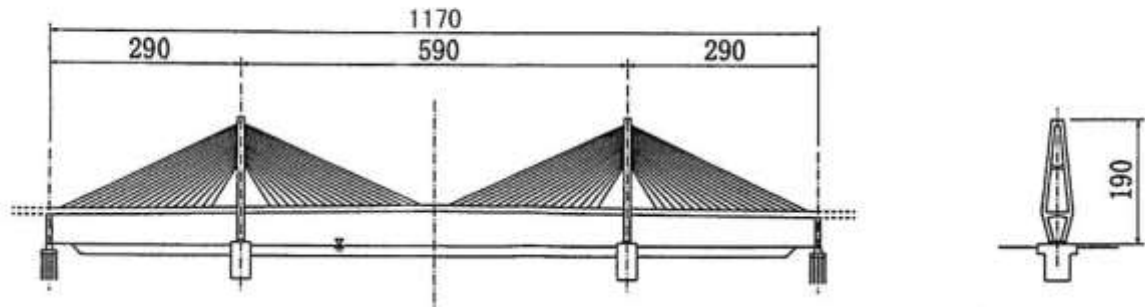
LSB20105,MEIKO-CHUOH,名港中央大橋
