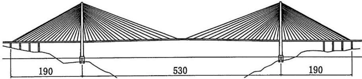
LSB20201,SKARNAUDET,
