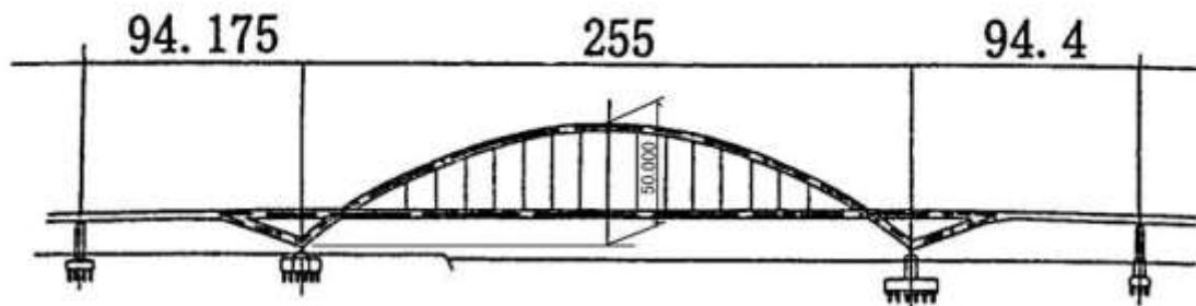
LSB30129,KISHIWADA,岸和田大橋
