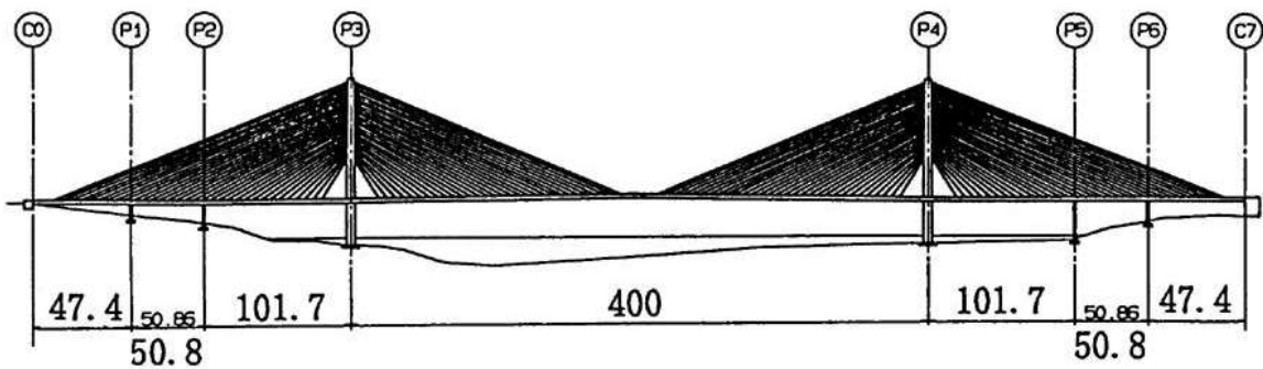
LSB20207,LE PONT SUR L'ELRON,
