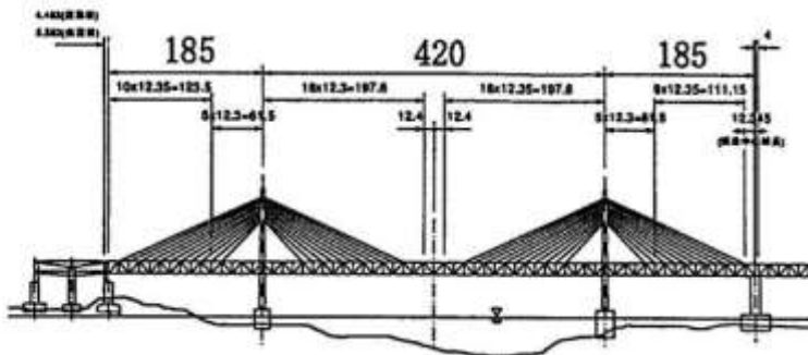
LSB20117, IWAKURO-JIMA, 岩黒島橋
