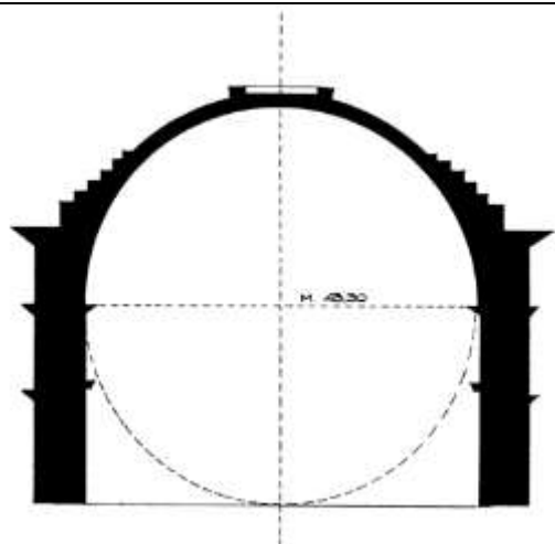
KWM022, パンテオン断面図
