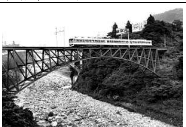
A20061、千垣橋梁、富山県、立山町～大山町、常願寺(じょうがんじ)川、富山地方鉄道/立山線、1932
