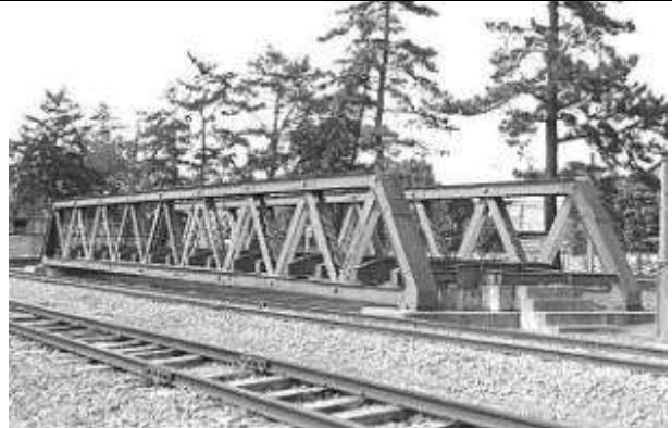
T40041、(六郷川橋梁)、静岡県、三島市、JR 東海三島職員研修センター(保存展示)、1965
