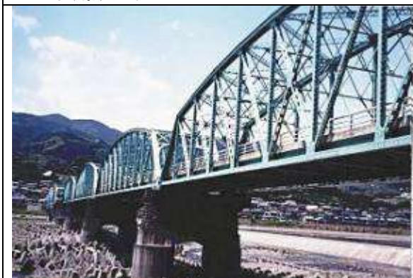
T80054、富士川橋、静岡県、富士市、富士川、国道1号、1924
