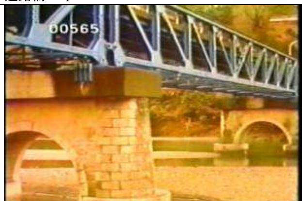
565、BBS9208201、秋葉橋、JP、静岡県、春野町、大正15年建設、トラス道路橋3、19??????
