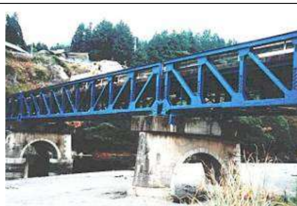
T80144、秋葉橋、静岡県、周智郡春野町、気田川、県道、1926
