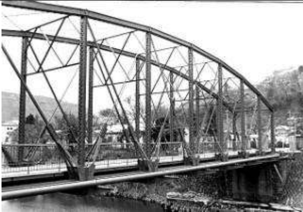
T30211、森村橋、静岡県、小山町、鮎沢川、富士紡績小山工場、1906
