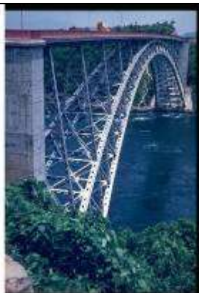
西海橋, JP, 大村湾, 鋼固定アーチ, 1961, 314m 戦後の長大橋の始め
