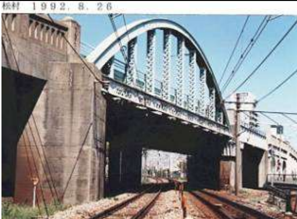
A50091、天神橋、兵庫県、神戸市須磨区天神町 1～天神 2、(山陽本線)、国道 2 号、1927
