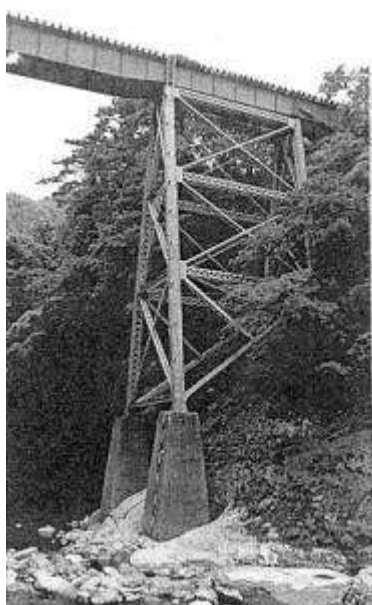
G40061、第十三米代川橋梁、秋田県、鹿角市、米代川、花輪線、1931
