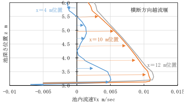
図-8 沈殿池上流・中央部流れ方向の流速 (横断方向越流堰 t = 4, 000sec)
