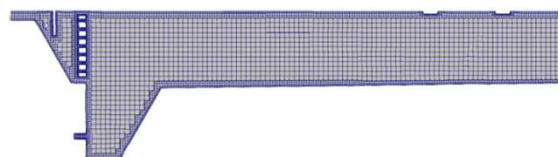
図-5 解析に利用したメッシュ
