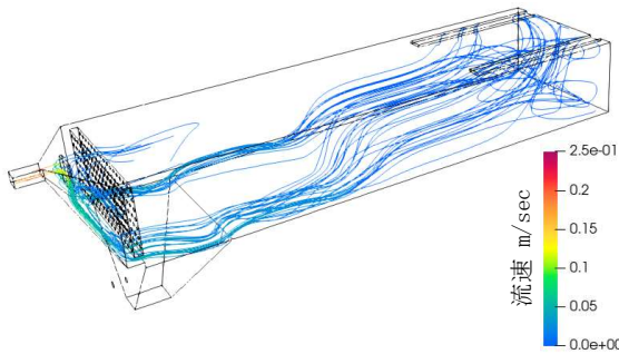
図-9 流入から越流堰に至る流線 ( t=1,000\text{ sec} ) 【越流堰配置：流れ方向】
