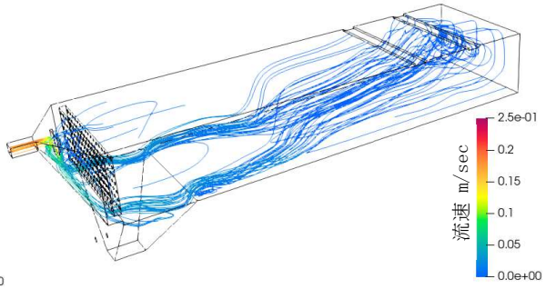
図-10 流入から越流堰に至る流線 ( t=1,000\text{ sec} ) 【越流堰配置：流れと直角方向】
