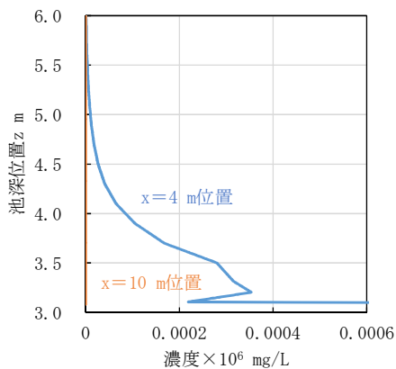
図-11 沈殿池上流から 4.0 、 10.0\text{m} 位置の中央部の濃度(縦断方向越流堰 t=5,000\text{sec} )
