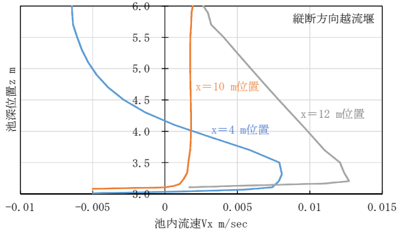
図-7 沈殿池上流・中央部流れ方向の流速 (縦断方向越流堰 t = 4, 000sec)
