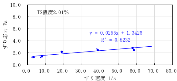
図-3 低濃度濃縮汚泥のずり速度とずり応力の関係
