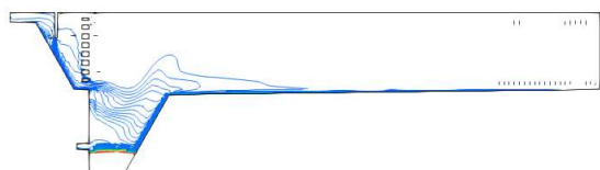
図-13 沈殿池内中央部の汚泥濃度分布 (縦断方向越流堰 t = 10,800 sec)
