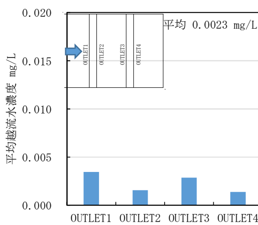
図-16 越流堰からの平均流出濃度 (処理水濃度 t = 10,800 sec)
