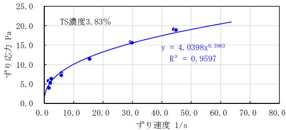
図-4 高濃度濃縮汚泥のずり速度とずり応力の関係
