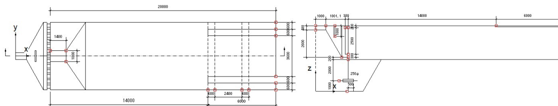
図-1 最終沈殿池形状と越流堰配置（縦断方向と横断方向）
