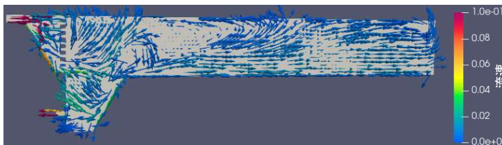
図-6 沈殿池内中央部の流向(縦断方向 t = 10,800\text{sec} )
