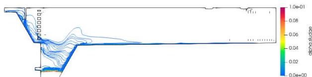
図-14 沈殿池内中央部の汚泥濃度分布 (横断方向越流堰 t = 10,800 sec)
