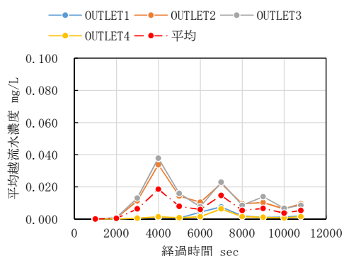
図-17 経過時間ごとの越流堰平均越流水濃度(縦断方向越流堰)
