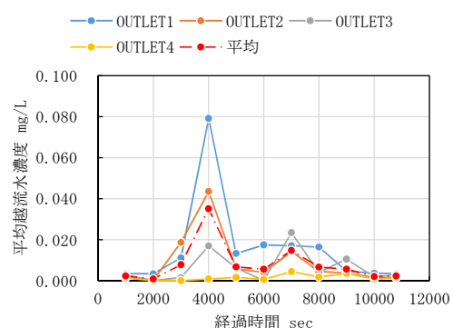
図-18 経過時間ごとの越流堰平均越流水濃度(横断方向越流堰)
