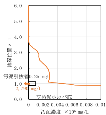
図-12 汚泥ホopp中央部の濃度(縦断方向越流堰 t=10,800\text{sec} )
