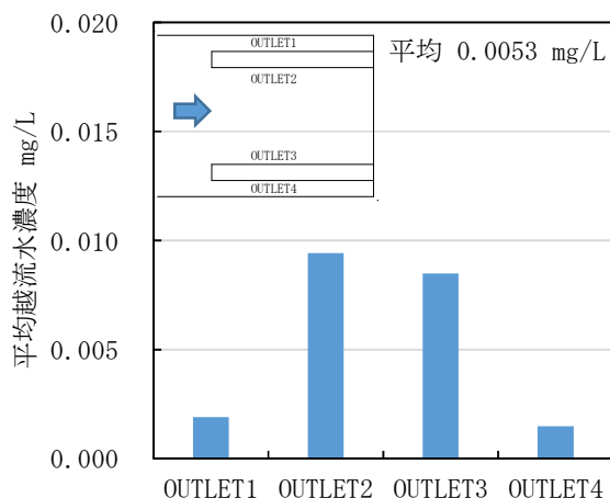
図-15 越流堰からの平均流出濃度 (処理水濃度 t = 10,800 sec)
